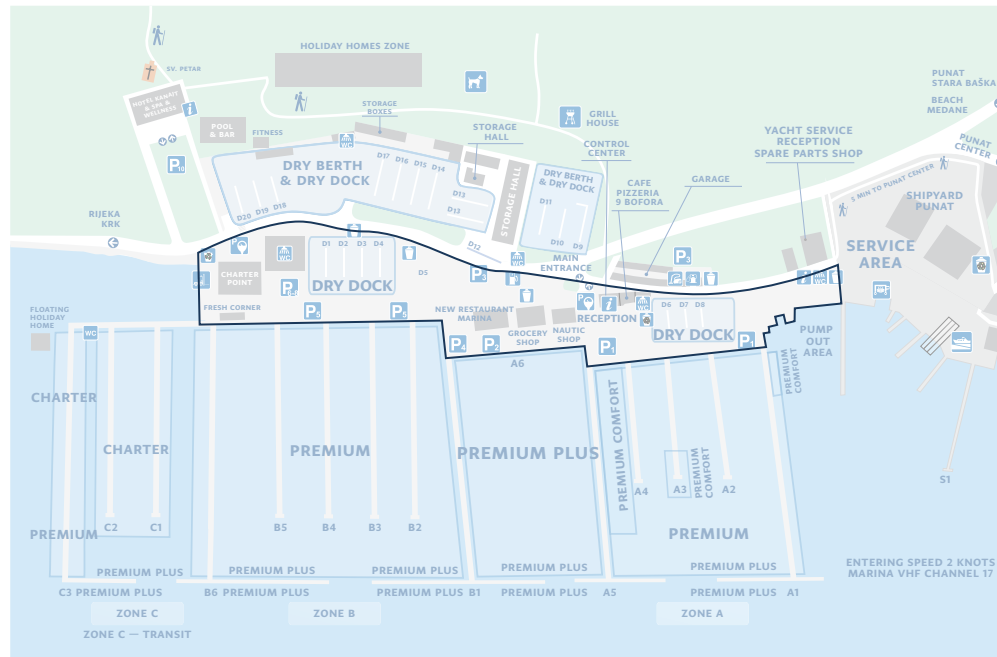
Priloga 1: Grafični prikaz suhe marine in luke v namenskem pristanišču—Marina Puntat
